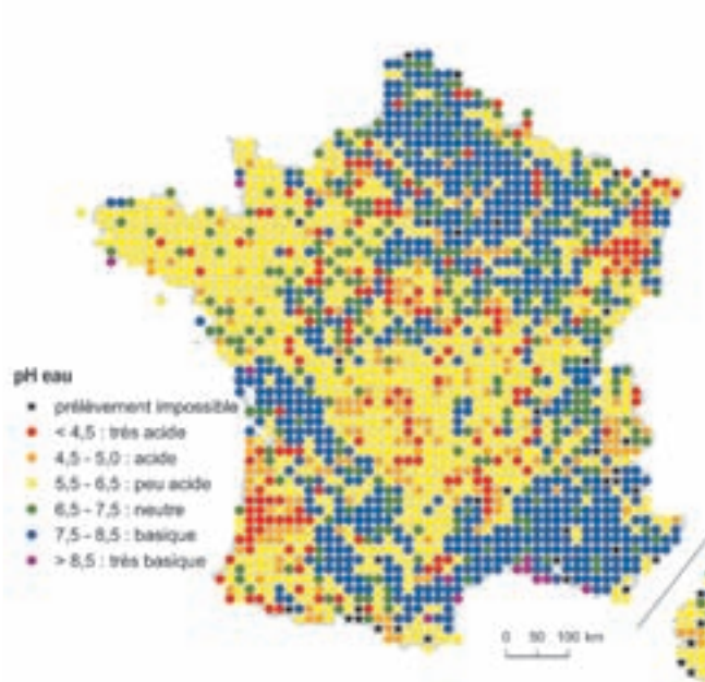
Le pH des horizons de surface des sols de France métropolitaine des sites du Réseau de Mesures de la Qualité des Sols (mesuré) et celui des sols forestiers (prédit par la végétation)
